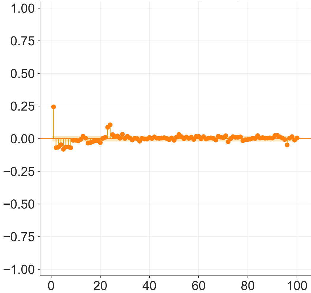
PACF MSM (2024)
